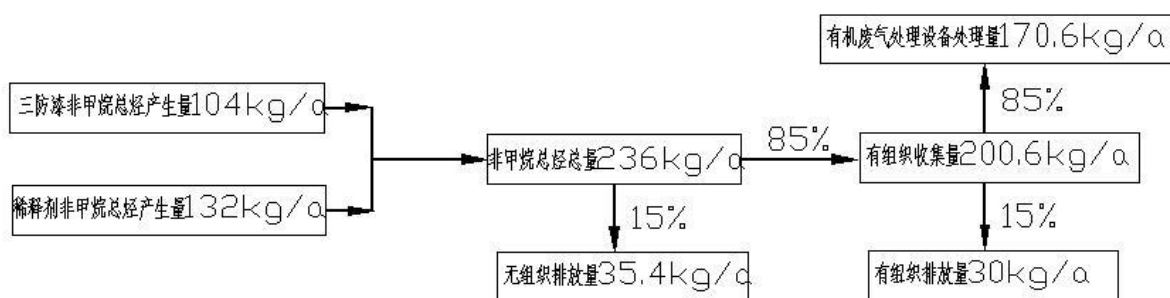
图6 A座DIP车间非甲烷总烃平衡图
