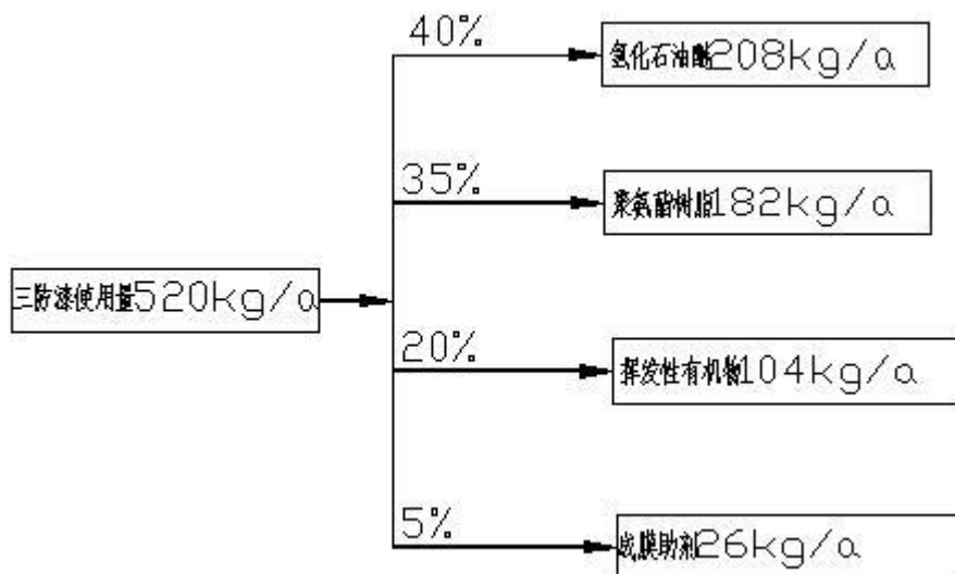
图4 B座生产车间三防漆平衡图（单位：m 3 /a）
