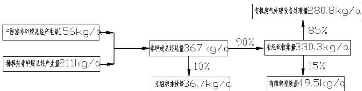
图 5 A 座 DIP 车间非甲烷总烃平衡图
