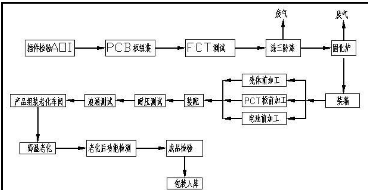
图3 智能采集终端生产工艺流程及产污环节分析图
