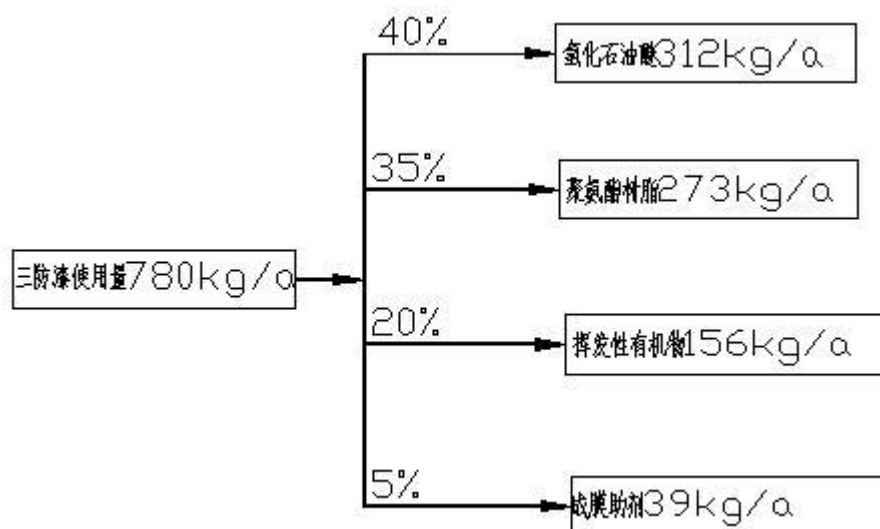
图 4 A 座生产车间三防漆平衡图（单位：m 3 /a）
