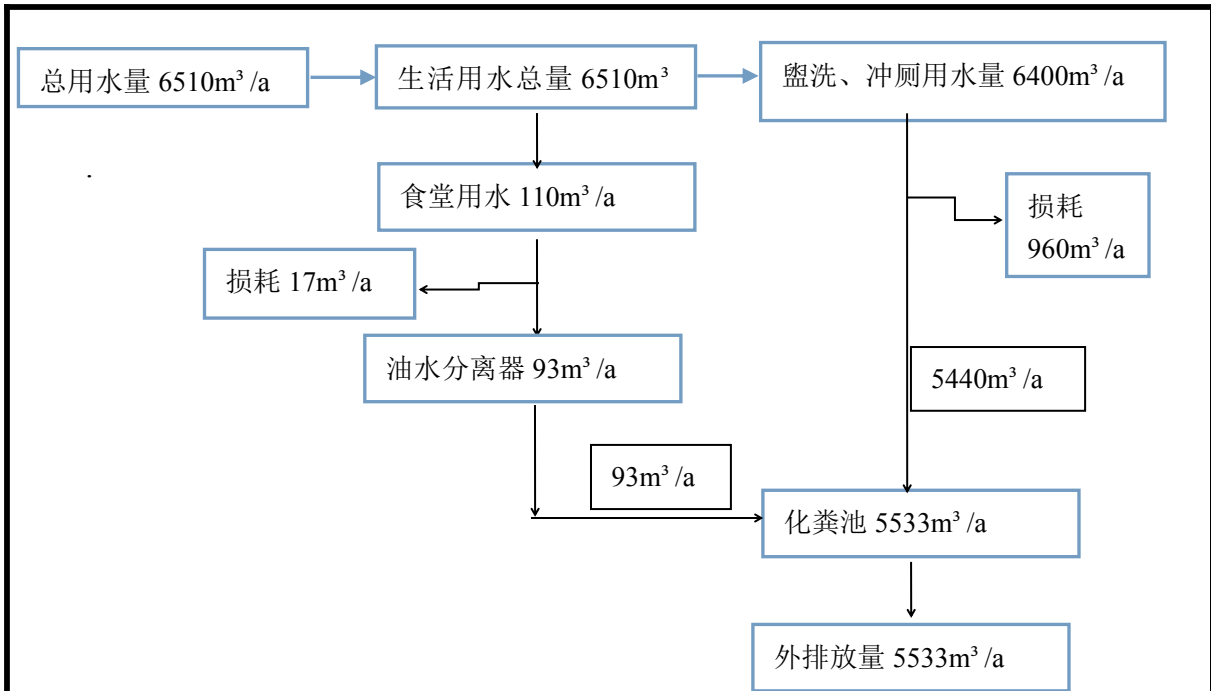
图 4 项目水平衡图（单位： \text{m}^3/\text{a} ）
