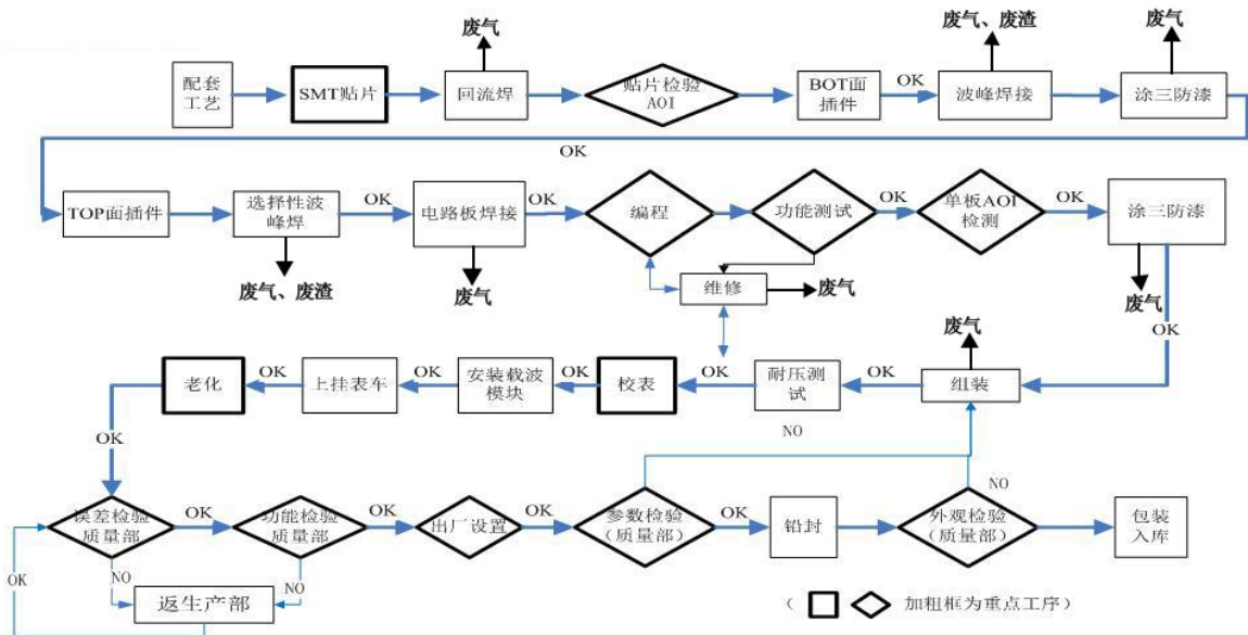
图 2 智能电表生产工艺流程及产污环节分析图
